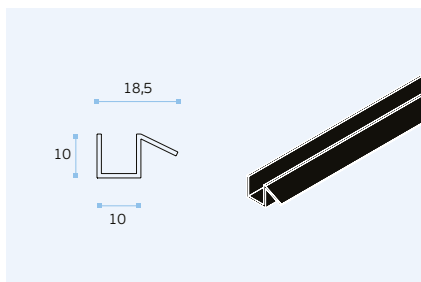
IN.15.996.J (2000mm) Vedante para vidro / PVC seals for glass / Sellos para cristal
