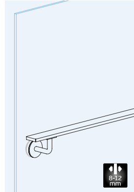
IN.18.136 Suportes de corrimão para vidro / Hand rail support for glass/ Soporte pasamanos para cristal.
